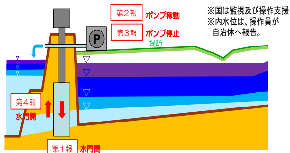
図 4-9 水門操作防災周知の連絡体制
