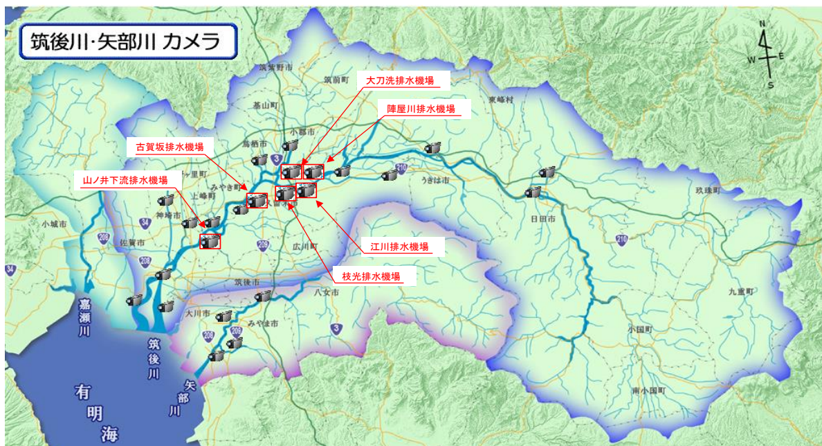
図 4-13 監視カメラの設置箇所
