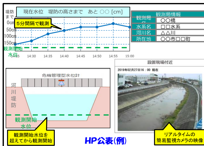
図 4-16 危機管理型水位計、監視カメラの設置例
