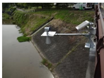
危機管理型水位計設置(例)
